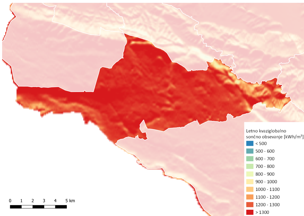
Slika 21: Povprečna letna energija kvaziglobalnega sončnega obsevanja površja na območju Občine Komen.
