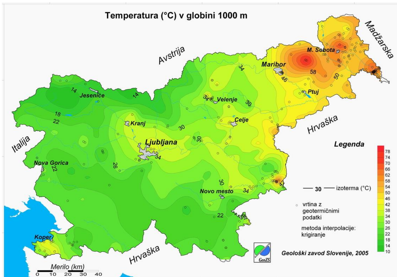
Slika 24: Karta temperature (°C) v globini 1000 m. Vir: Geološki zavod Slovenije.
