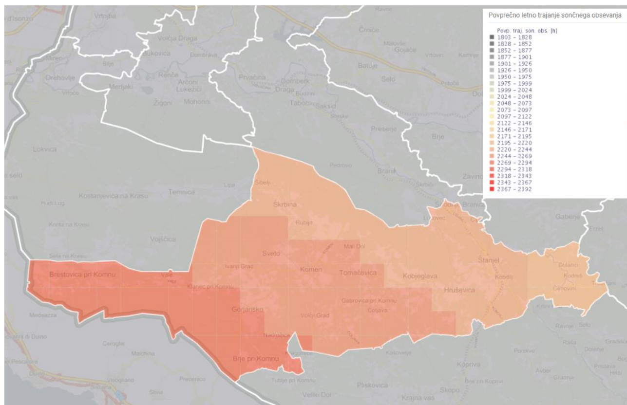
Slika 20: Povprečno trajanje sončnega obsevanja (ure) v obdobju 1981 – 2010 v Občini Komen.
