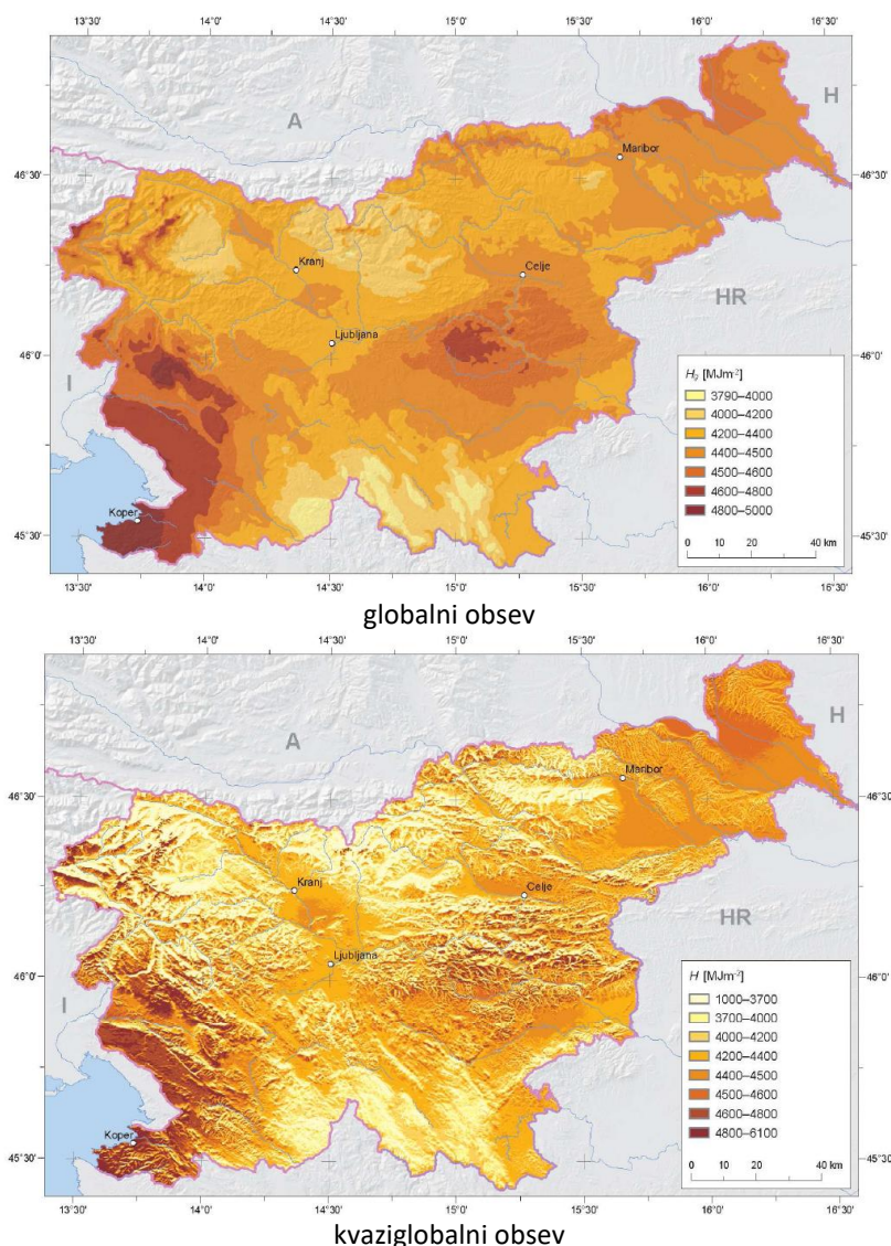
Slika 19: Letni globalni in kvaziglobalni obsev v Sloveniji. Vir: Sončna energija v Sloveniji, Jože Rakovec, Damijana Kastelec in Klemen Zakšek.
