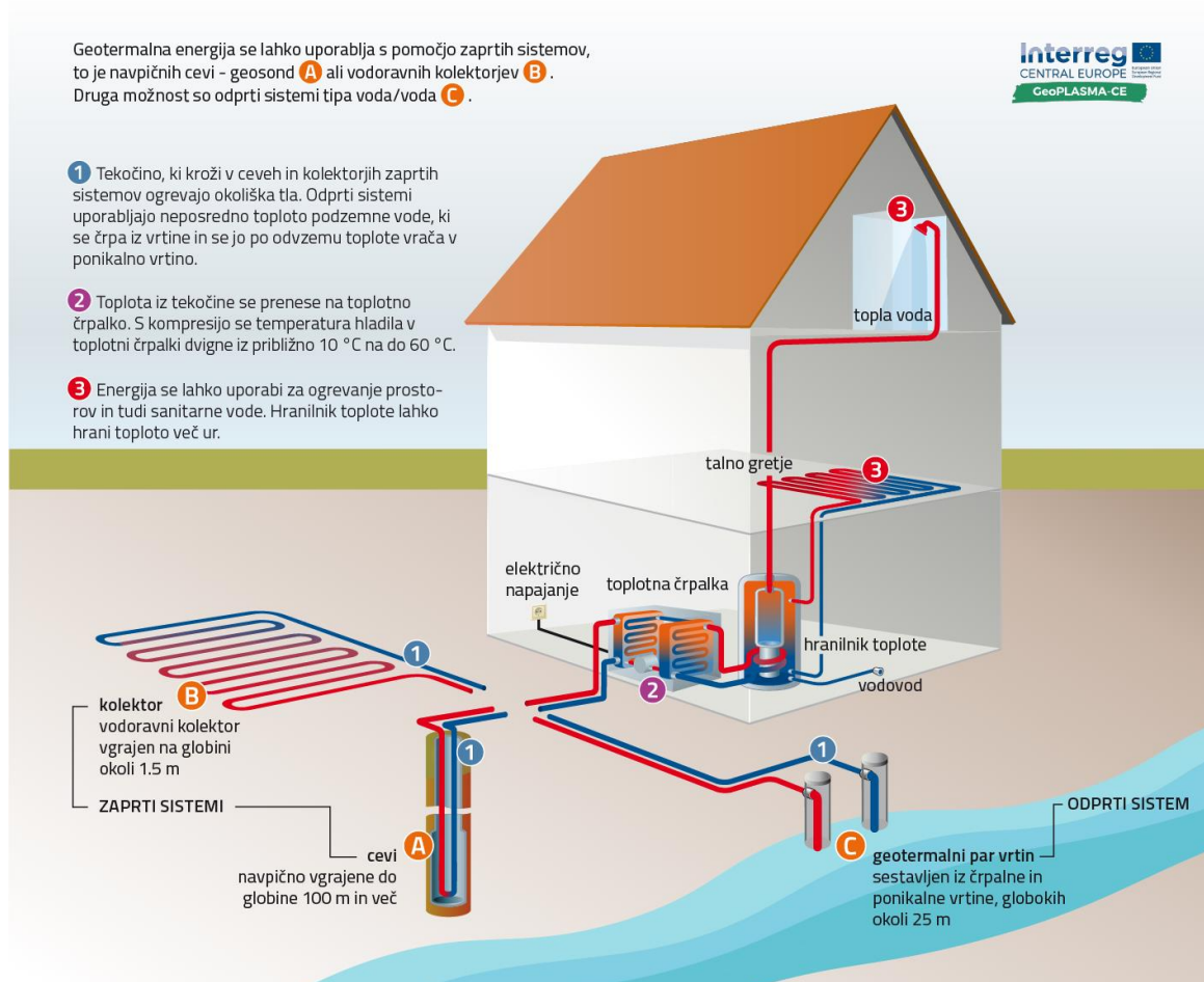
Slika 23: Shematski prikaz delovanja zaprtega in odprtega sistema za izrabo plitve geotermalne energije.
