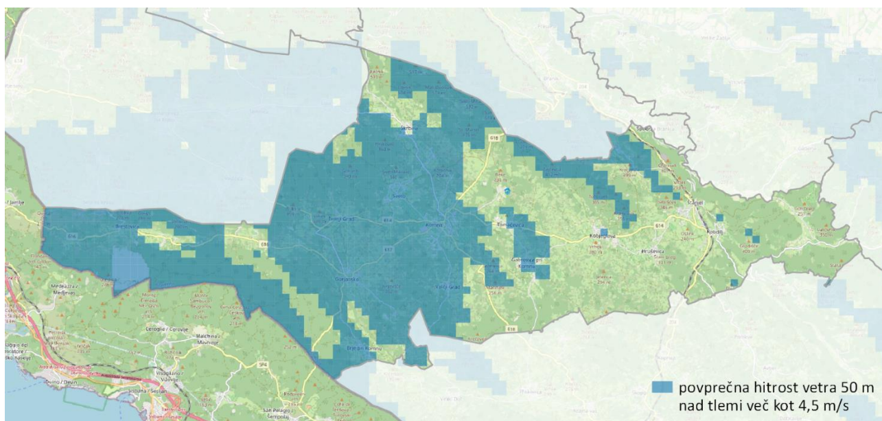
Slika 33: Območja v Občini Komen, kjer ocenjena povprečna letna hitrost vetra 50 m nad tlemi presega hitrost 4,5 m/s. Vir podatkov: Global Wind Atlas, GURS; vir kartografske podlage: OSM.
