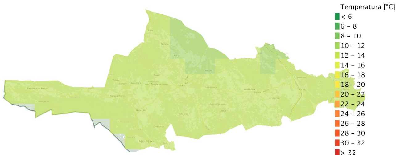
Slika 25: Temperatura v globini 100 m na območju Občine Komen.
