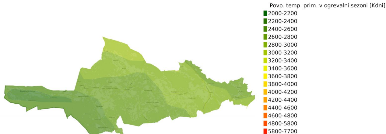
Slika 7: Povprečni temperaturni primanjkljaj (Kdan) 1971-2001 v Občini Komen.
