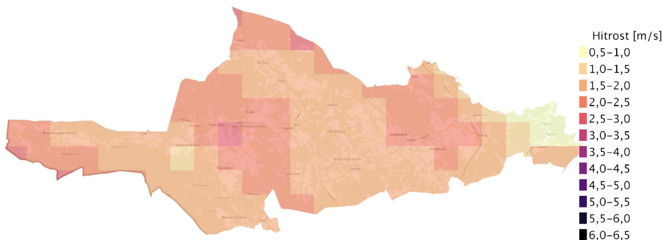
Slika 29: Povprečna letna hitrost vetra 10 m nad tlemi v obdobju 1994-2000 na območju Občine Komen na podlagi modela Aladin DADA. Vir podatkov: ARSO, kartografija Monolit d. o. o.
