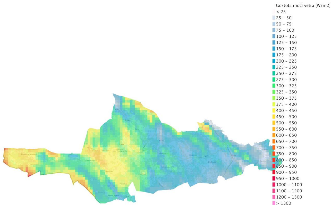
Slika 31: Ocenjena povprečna letna gostota moči vetra 50 m nad tlemi na območju Občine Komen na podlagi podatkov Svetovnega vetrnega atlasa (Global Wind Atlas). Vir: Global Wind Atlas, kartografija Monolit d.o.o.
