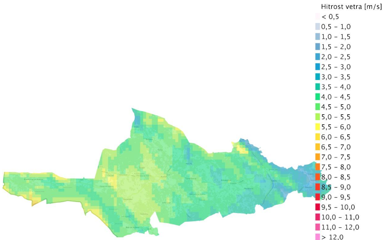
Slika 30: Ocenjena povprečna letna hitrost vetra 50 m nad tlemi na območju Občine Komen na podlagi podatkov Svetovnega vetrnega atlasa (Global Wind Atlas). Vir podatkov: Global Wind Atlas, kartografija Monolit d. o. o.
