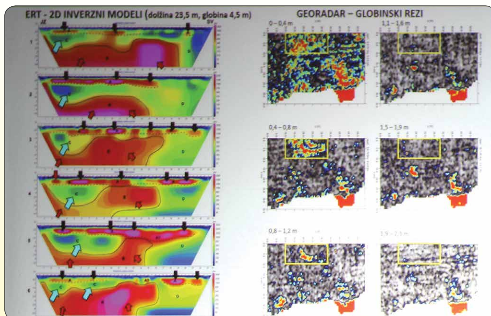
Ponazoritev georadarskih meritev.
