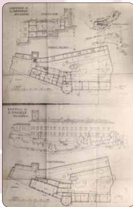
Fabianijevi načrti za obnovo štanjelskega gradu iz tridesetih let 20. stoletja. Grad Štanjel, v katerem so med I. svet. vojno bivali avstrijski vojaki, je Maks Fabiani, štanjelski župan med 1935 in 1945, obnovil in preuredil v center občine z uradi, osnovno šolo, otroškimi vrtcem, ambulanto, kinodvorano.
