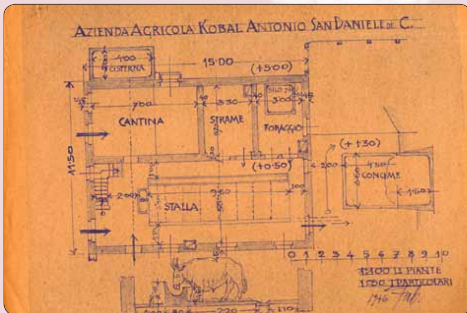
Fabianijevi načrti za novo domačijo Kobal v dolnjem Štanjelu iz leta 1946. Družina je imela v lasti hišo v gornjem Štanjelu, ki je bila med vojno močno poškodovana. Zavezniško vojaško upravo v Trstu so zaprosili za financiranje gradnje nove stavbe v vrednosti, ki je bila ocenjena za obnovo stare.
