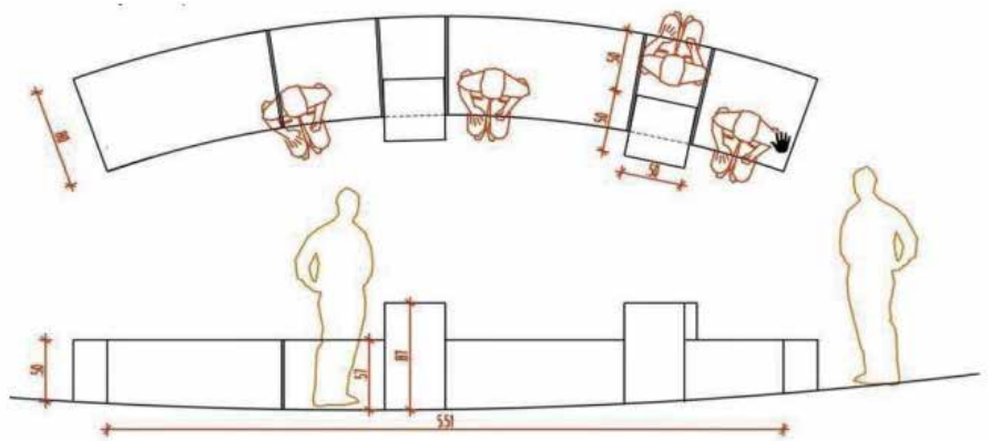
Shema kamnite klopi na Gledanici (N. Kolenc, december 2019).
